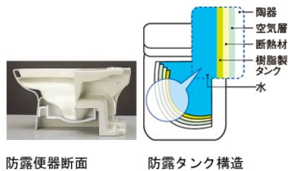
防露便器断面
